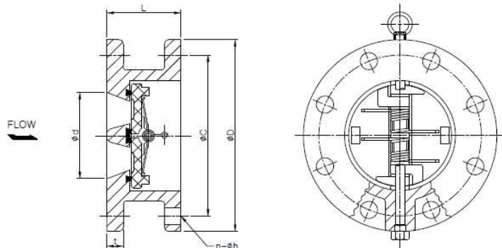
FLANGE
